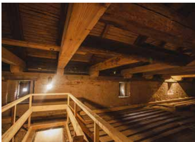
Atjaunotas pirmā un otrā stāva pārseguma sijas. The joist frames of the first and second floor are restored.
